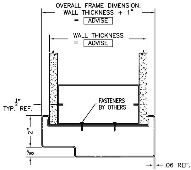
JAMB PROFILE, WRAPPING S/S FRAME
